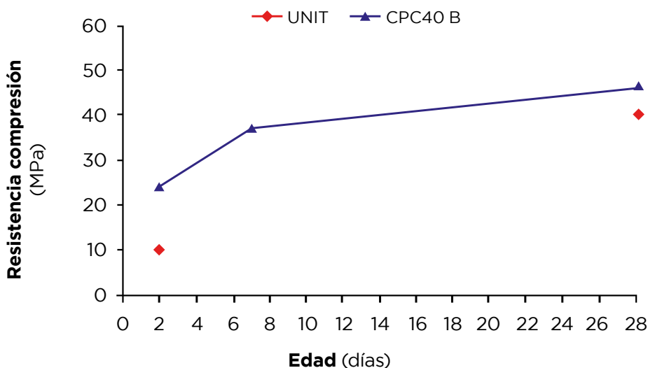
Fig. 1 - Resistencia a compresión del mortero UNIT ISO 679
